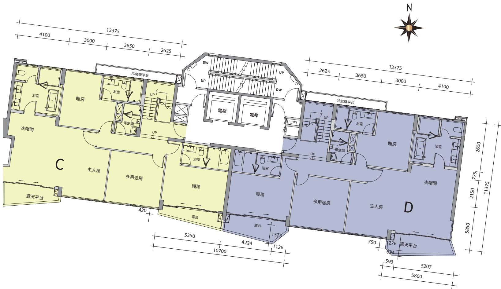
座向圖 Block Plan
